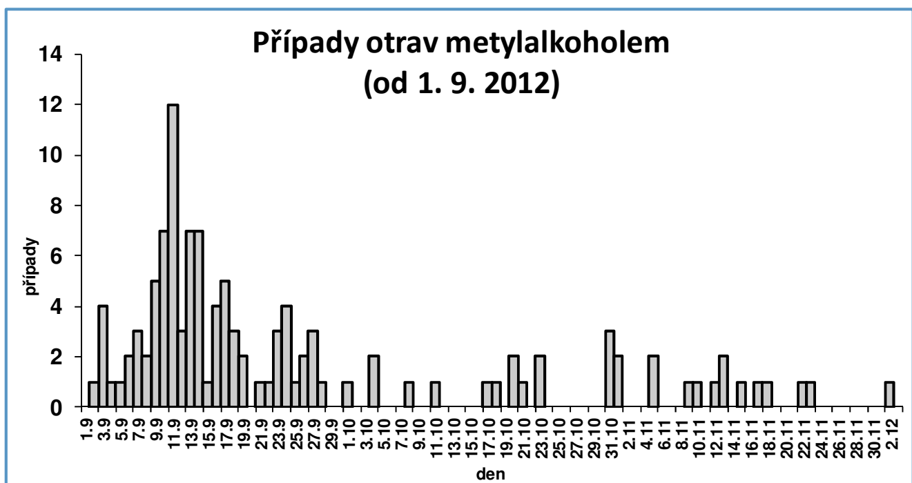
Graf 4: Případy otrav metylalkoholem od 1. 9. 2012 v ČR
