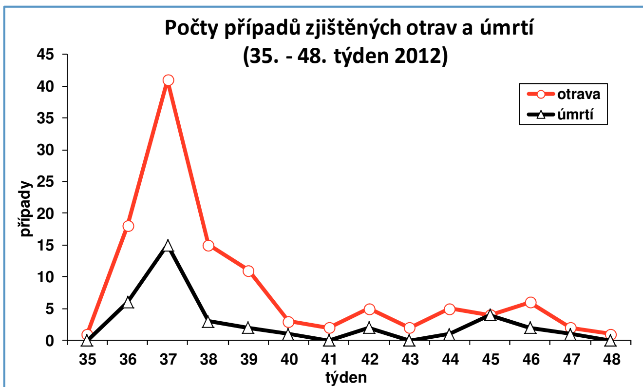
Graf 2: Počty případů zjištěných otrav a úmrtí v ČR od 35. do 48. týdne
