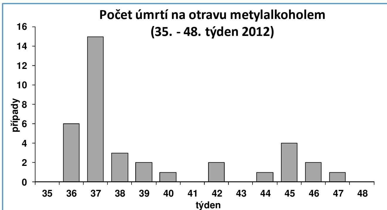
Graf 3: Počet úmrtí na otravu metylalkoholem v ČR od 35. do 48. týdne
