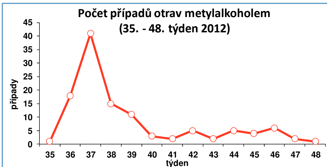
Graf 1: Počet případů otrav metylalkoholem v ČR od 35. do 48. týdne
